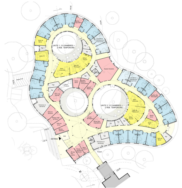
Plan Rez-de-Chaussée 1/200
